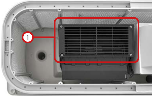
Fig. 6.3.4.11 Blower B 600
